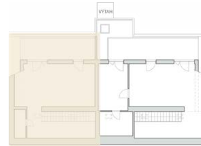
6. Nadzemní podlaží
